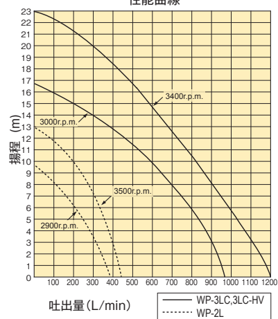
性能曲線
